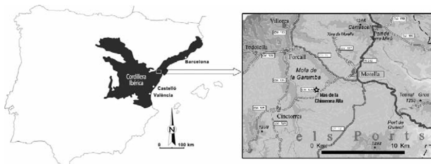
Fig. 1.- Localización geográfica del yacimiento del Mas de la Chimenea Alta, Morella (Castellón).
