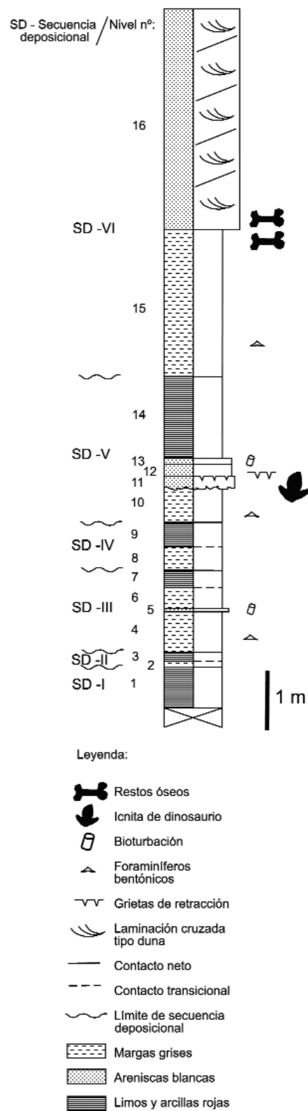
Fig. 2.- Columna estratigráfica de los materiales de la Formación Arcillas de Morella en el Mas de la Chimenea Alta.
