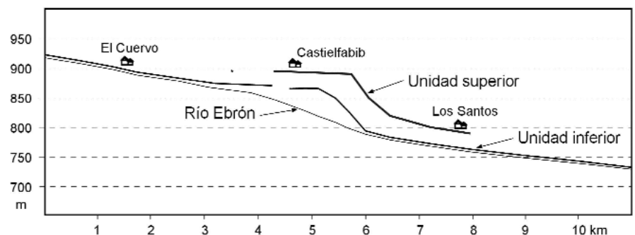
Fig. 4.- Perfiles longitudinales del río, unidad tobácea superior y unidad tobácea inferior.
