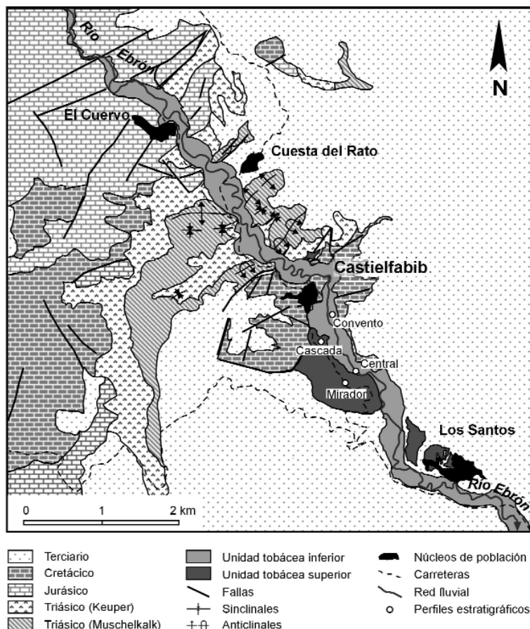
Fig. 2.- Mapa geológico y posición de los perfiles estratigráficos. Fig. 2.- Geologic map and location of studied stratigraphic sections.
