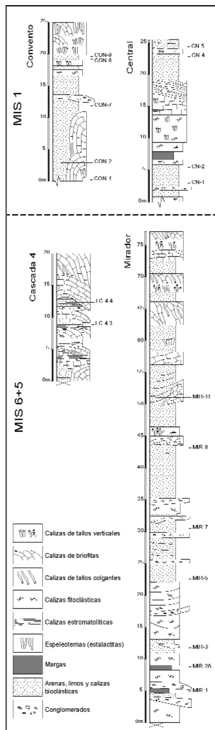
Fig. 5.- Perfiles estratigráficos sintéticos. Fig. 5.- Summarized stratigraphic sections.
