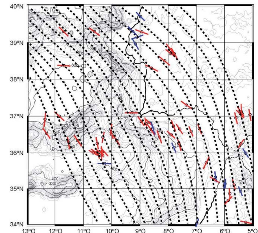
Fig. 2.- Direcciones de S_H para mecanismos de desgarre e inversos (líneas rojas) y para mecanismos focales de tipo normal (líneas azules).
