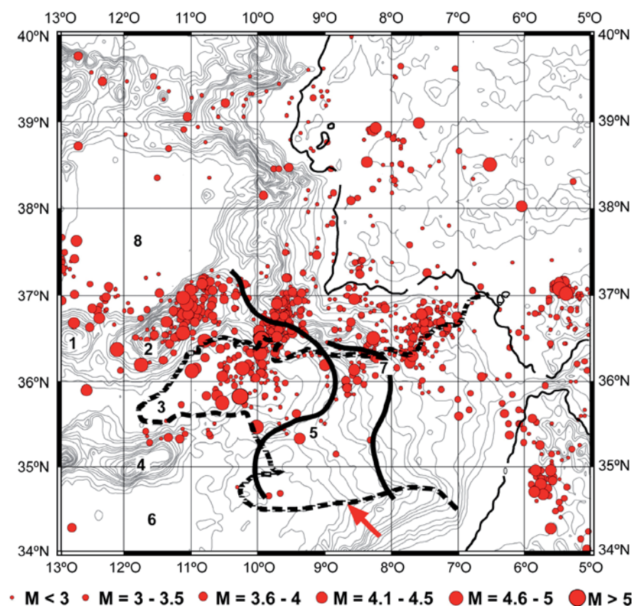
Fig. 1.- Sismicidad en el Golfo de Cádiz y áreas adyacentes para el periodo 2004-2010. M: Magnitud de los terremotos. Línea discontinua gruesa: Unidad Alóctona del Golfo de Cádiz. Las líneas continuas gruesas delimitan la litosfera de características transicionales entre oceánica (al oeste) y continental (al este y norte), según Medialdea (2004). 1: Relieve Hironnelle; 2: Banco de Goringe; 3: Llanura abisal de La Herradura; 4: Monte Coral Patch; 5: Cresta Coral Patch; 6: Llanura abisal del Sena; 7: Banco del Guadalquivir; 8: Llanura abisal del Tajo. La flecha indica la dirección de movimiento relativo de la placa africana con respecto a la placa euroasiática.
