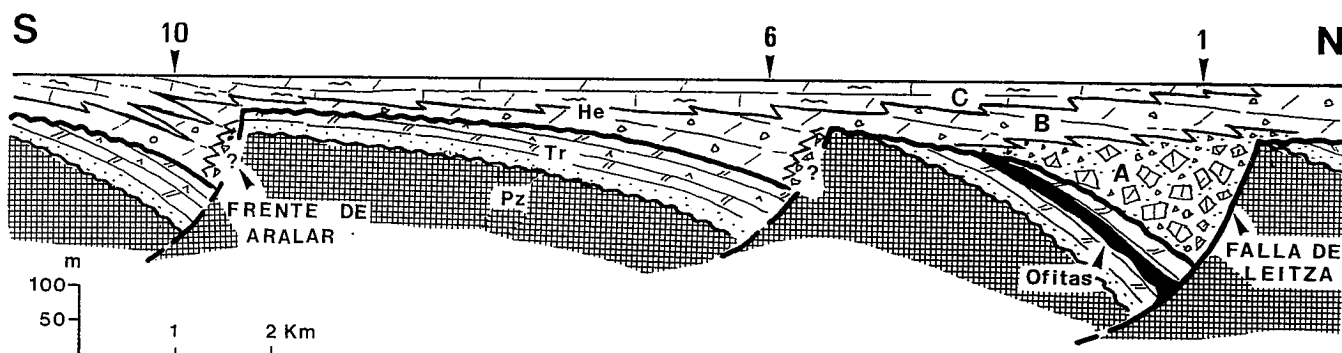
Fig. 3.— Sección transversal a la cuenca en la que se muestra la distribución de facies durante el Hettangiense (ver Fig. 1 para su localización; los números de la parte superior corresponden a los perfiles de referencia). Pz: Paleozoico, Tr: Triásico, He: Hettangiense. Facies (Hettangiense): A: Brechas y ruditas, B: Dolomías masivas y brechas, C: Calizas dolomíticas y dolomías.
